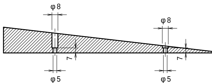
S1-S1断面図 (1/3)
